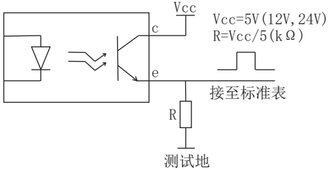
电能脉冲测试示意图
